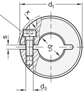
Zylinderschraube DIN 912
