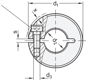
Zylinderschraube DIN 912
