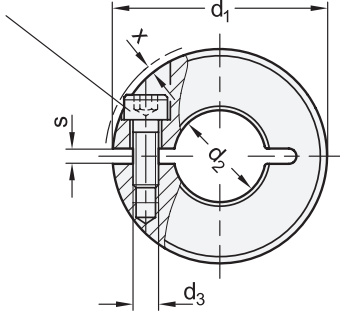
Zylinderschraube DIN 912
