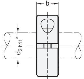
* empfohlene Durchmessertoleranz
